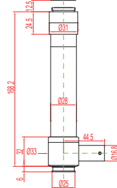
MTDP30C
