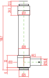
MTDP60C
