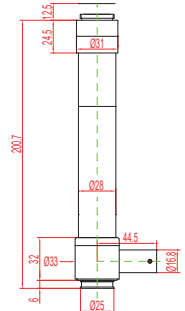
MTDP80C
